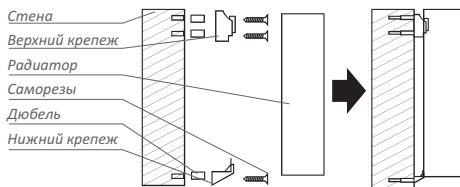
Рис. 11 Схема сборки настенного крепежа
