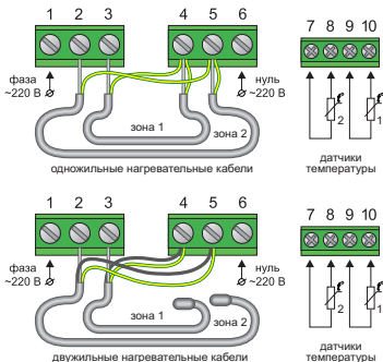
Рис. 7 Схема подключения к двухпроводной электрической сети
