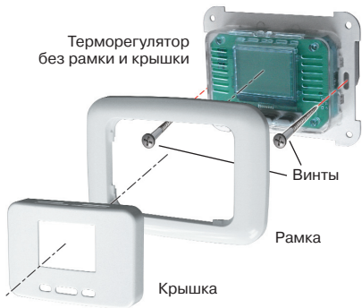
Рис. 10 Установка терморегулятора
