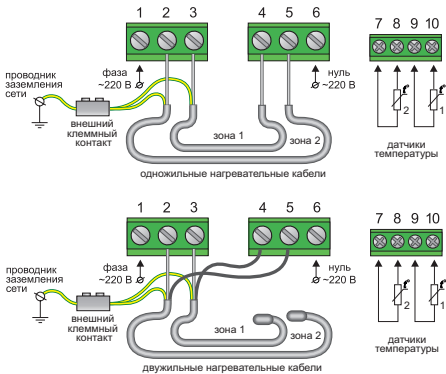
Рис. 8 Схема подключения к трехпроводной электрической сети
